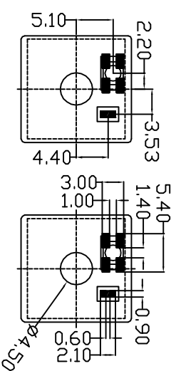
PCB板零件定位图
